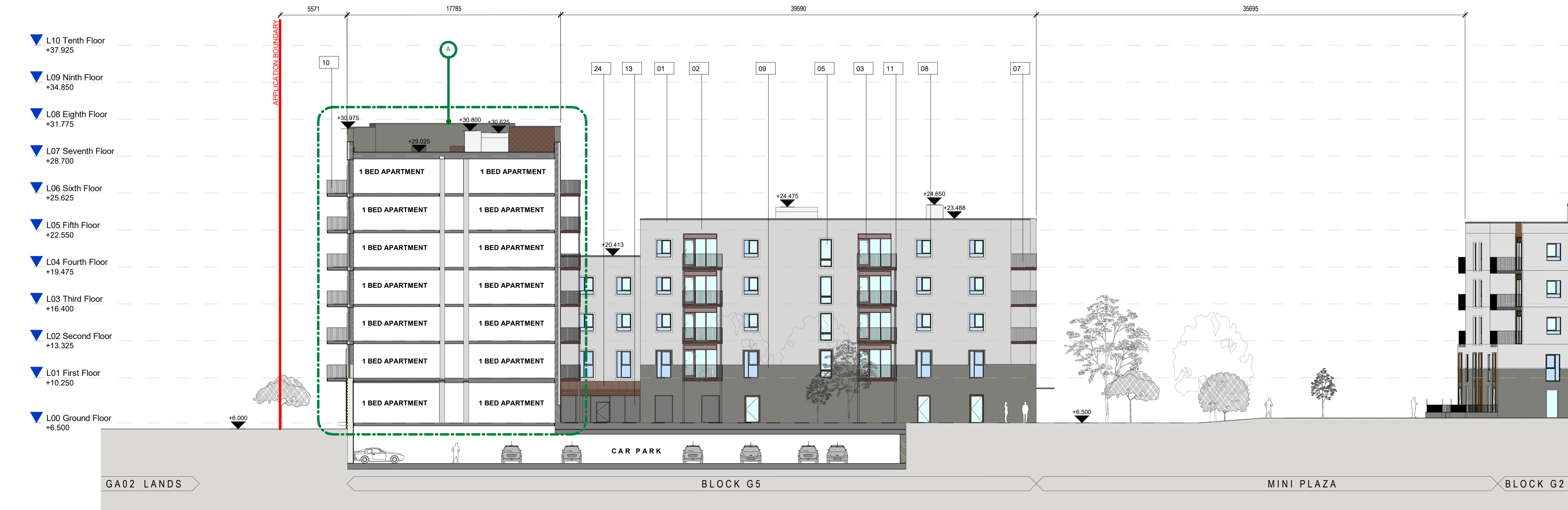
SECTION / ELEVATION DD 2 1:200
