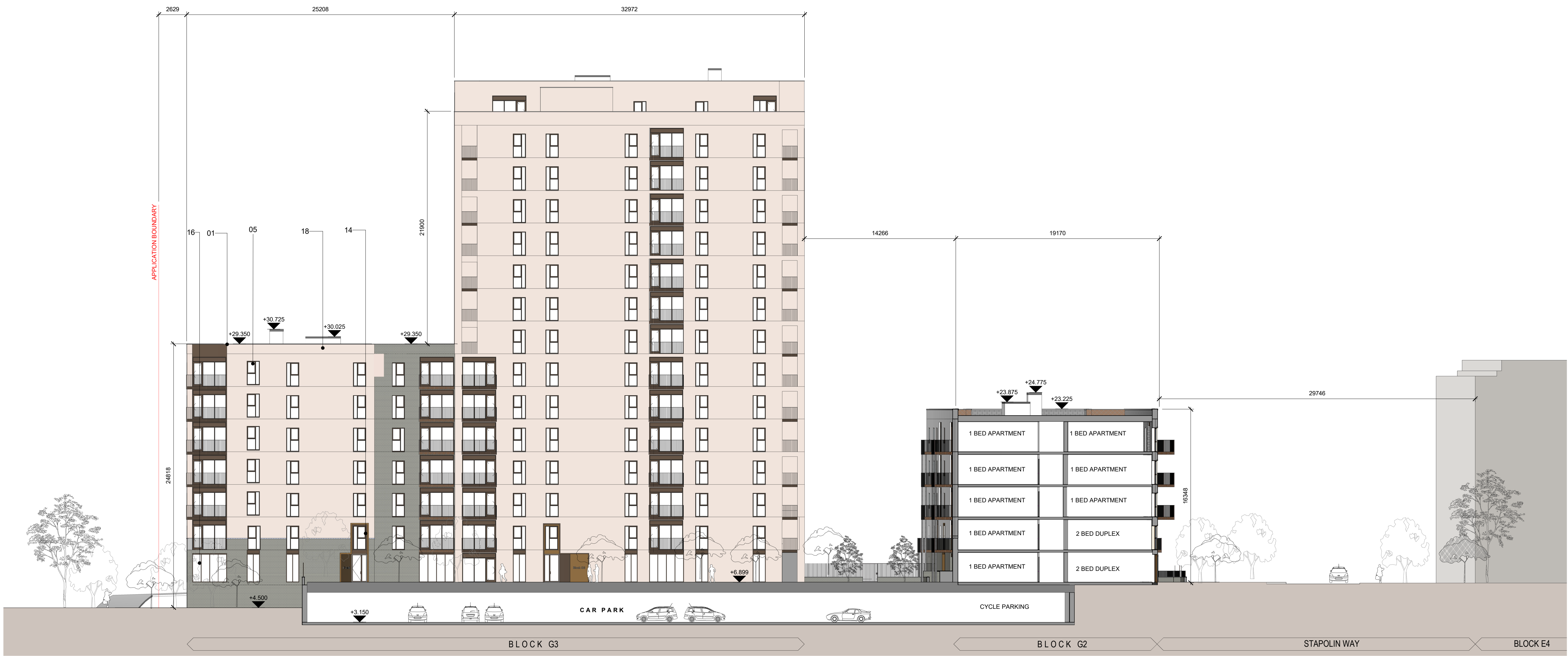
2 Section / Elevation DD 1:200
